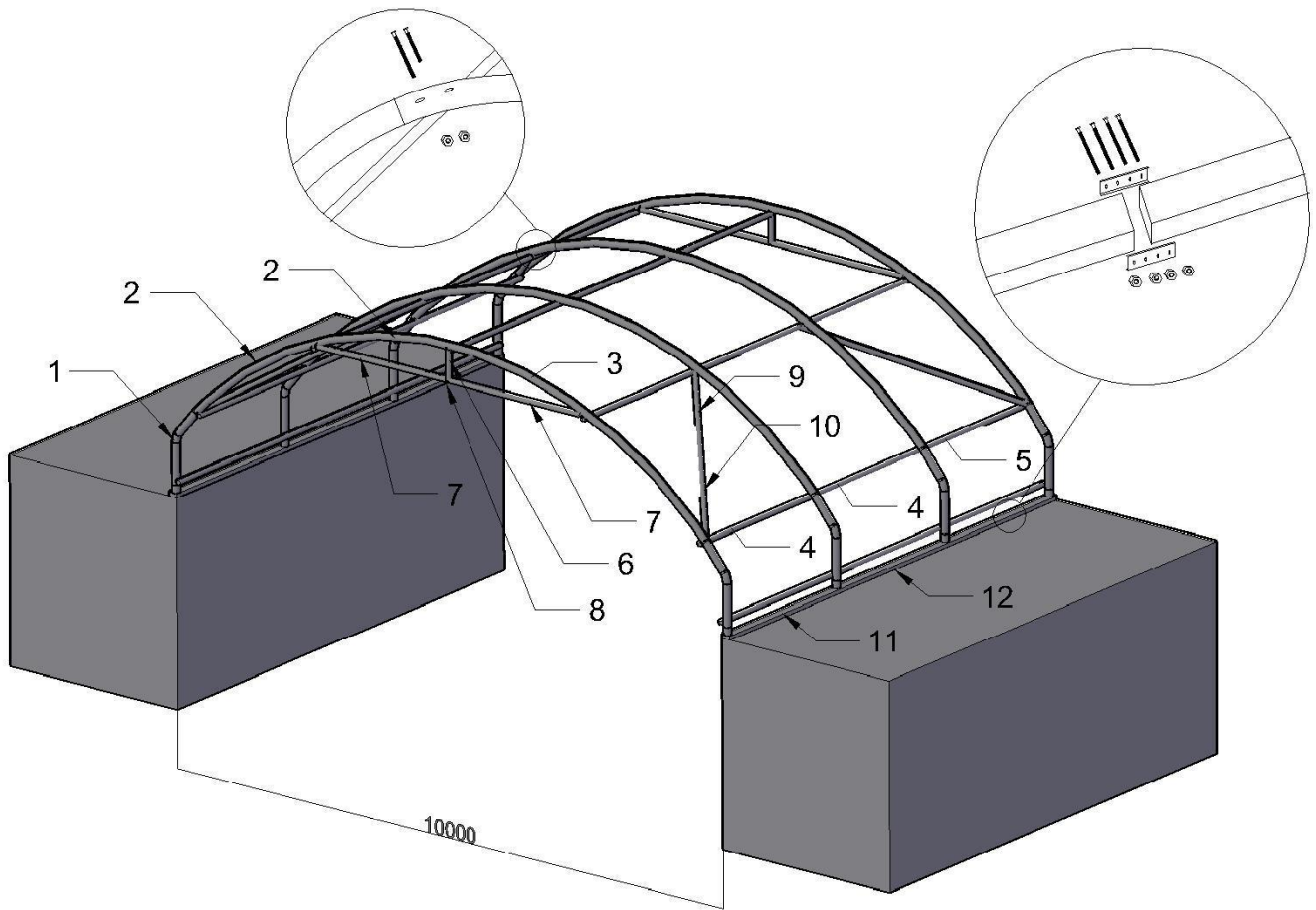
Door Frame Part List
